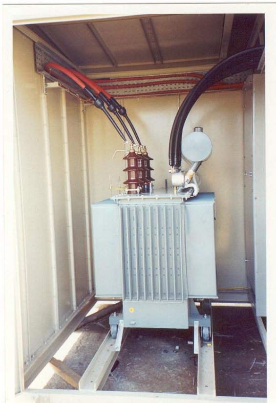
Εγκατάσταση υποσταθμού Εγνατίας
