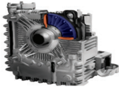
Σχήμα 2.22. Υδραυλικός επιβραδυντής
