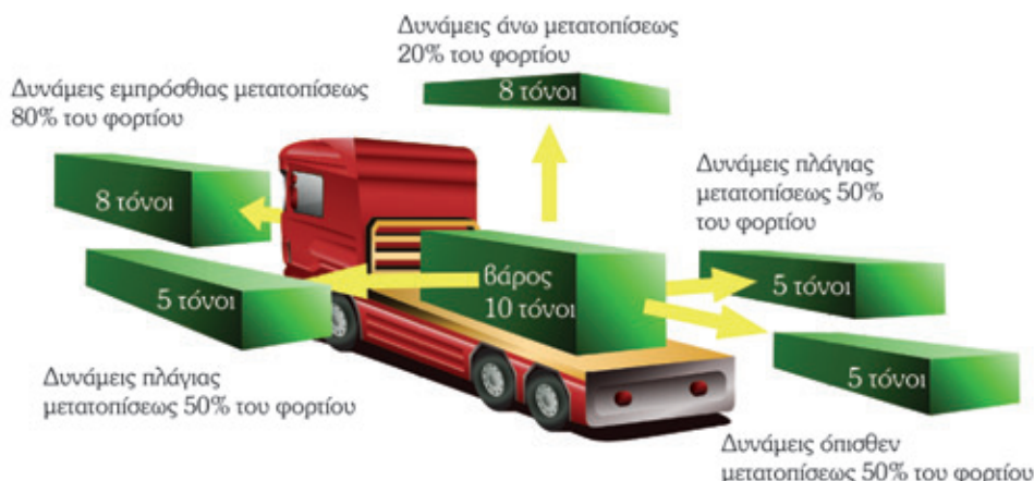
Σχήμα 2.29. Αναπτυσσόμενες δυνάμεις
