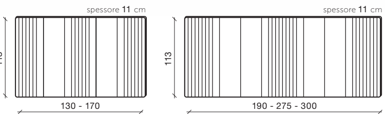
TESTATA PARETE
