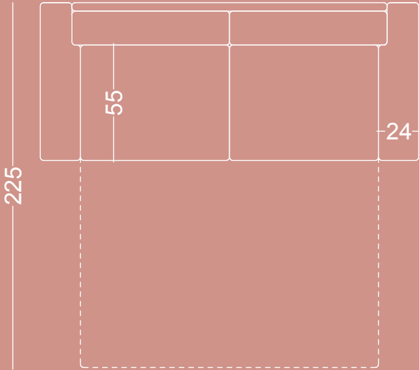
DIVANO APERTO
