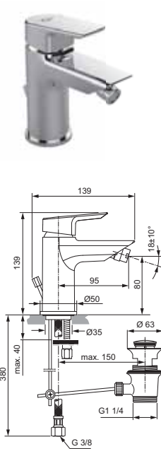
Tesi Bidet Mixer BC979AA
