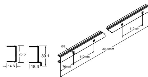
272-263 / 272-276 Βάση πείρου περιστροφής περσίδων Base profile for rotation louver 2050-602 (3m)
