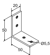
272-262 / 272-275 Βάση πείρου περιστροφής περσίδων Base profile for rotation louver 2050-607 (3m)
