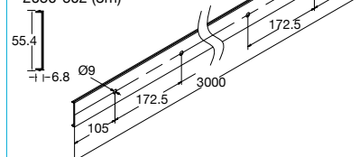
272-278 (από καπάκι/cover 2050-1K2) Βάση πείρου περιστροφής περσίδων Base profile for rotation of louver 2050-602 (3m)
