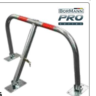
BPP2496 Μπάρα στάθμευσης • Αρθρωτή τύπου U • Διαστάσεις 70x45cm • Διάμετρος σωλήνα ø3,2cm 070924 49€
